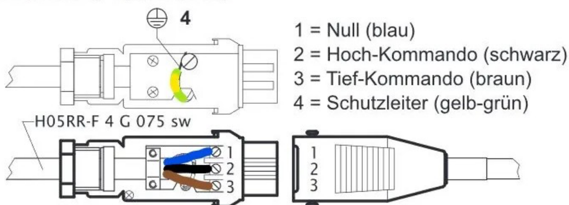
Anschlussplan Steckerkupplung bei Standard Motor
