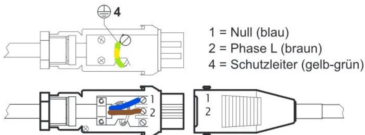
Anschlussplan Steckerkupplung bei Funk Motor
